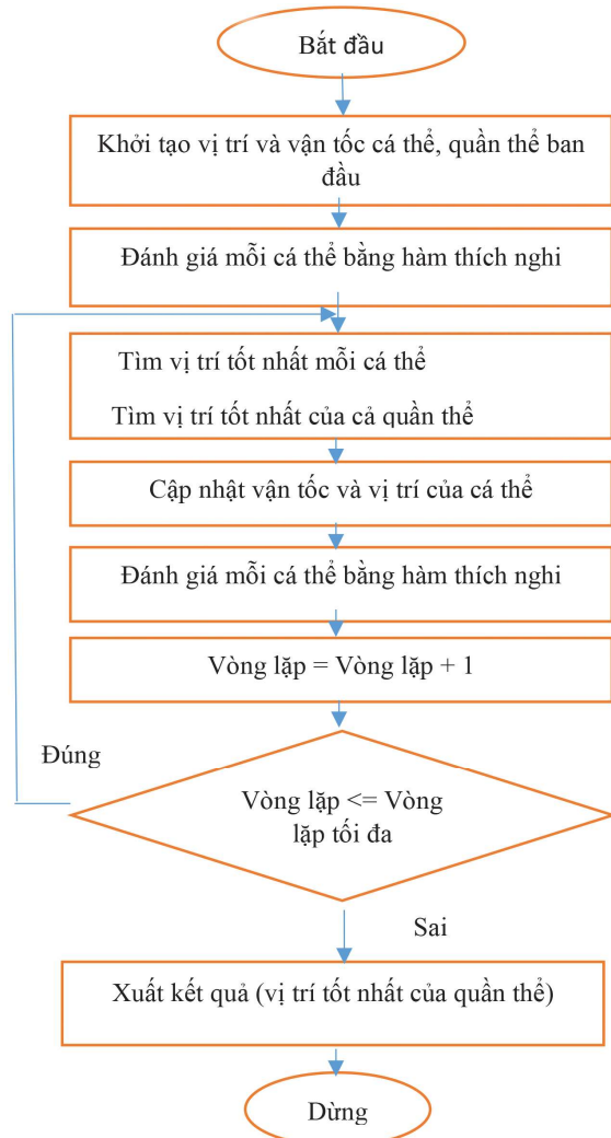
Hình 2.2: Sơ đồ thuật toán PSO tìm vị trí tối ưu
