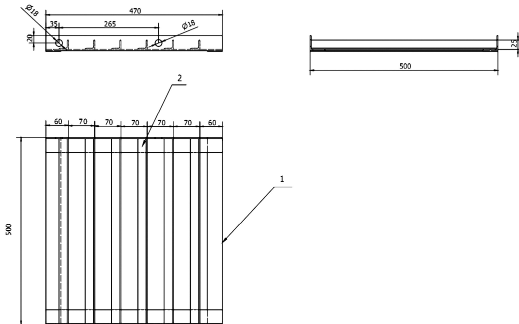
Hình 3. Khung sàng
