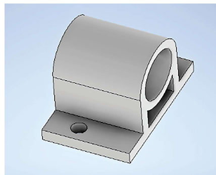
Hình 8. Thanh trượt đai ốc chống rơi
