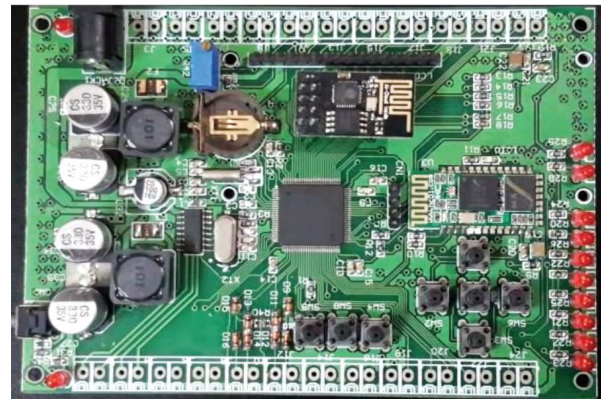
Hình 9. Board mạch hoàn thành
