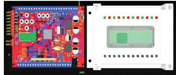
Hình 6. Board mạch 3D sau khi hoàn thành
