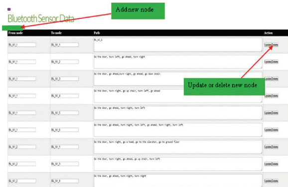
Hình 8. Giao diện quản lý trên hệ thống server
